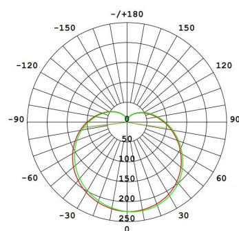
CURVA FOTOMETRICA
